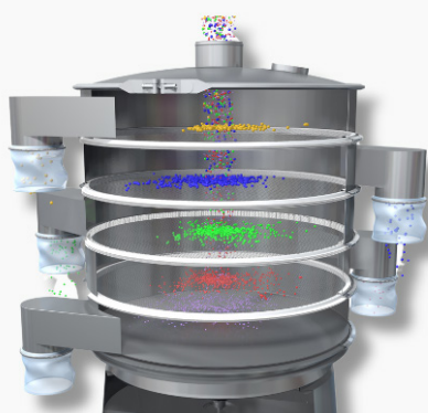
Finex Separator™ 一次筛分可同时处理5级物料
